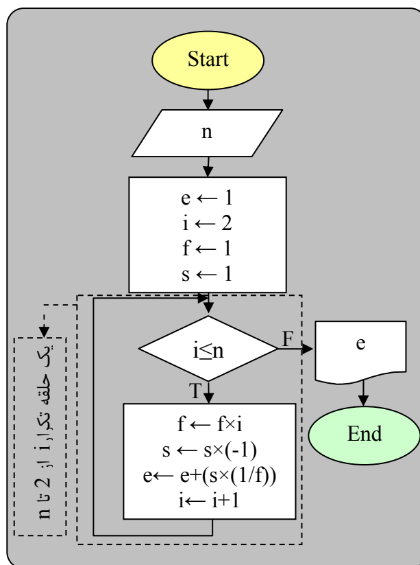
شکل ۲۰: فلوجارت مثال ۹
