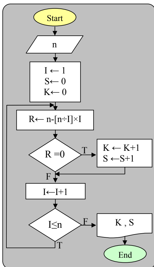
شکل ۱۶: فلوجارت مثال ۷
