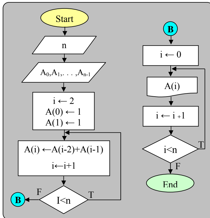
شکل ۲۵: فلوچارت مثال ۱۴
