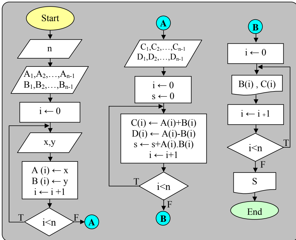
شکل ۲۴: فلوچارت مثال ۱۳
