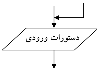
شکل ۹: نماد ورودی
