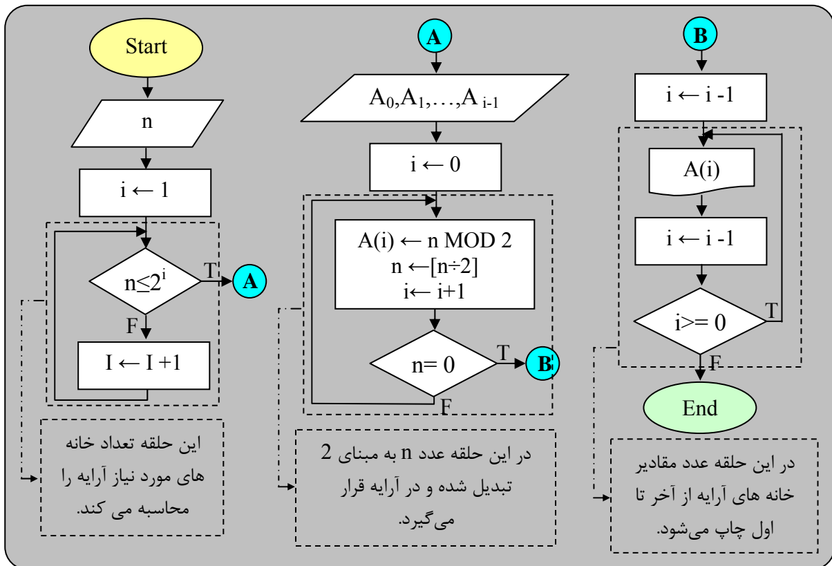
شکل ۲۳: فلوجارت مثال ۱۲
