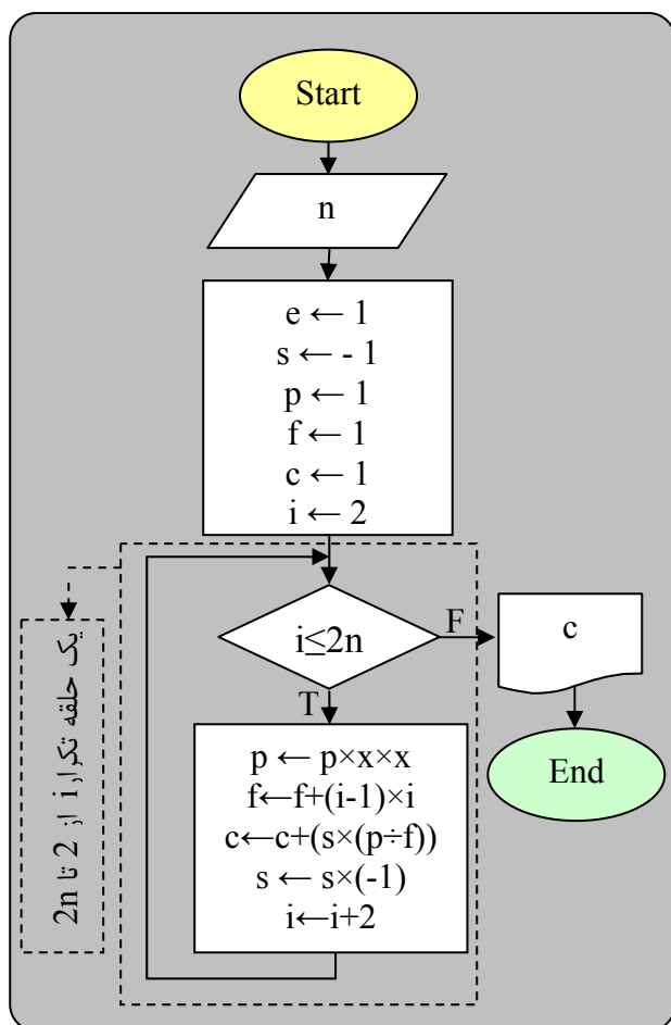
شکل ۲۱: فلوجارت مثال ۱۰
