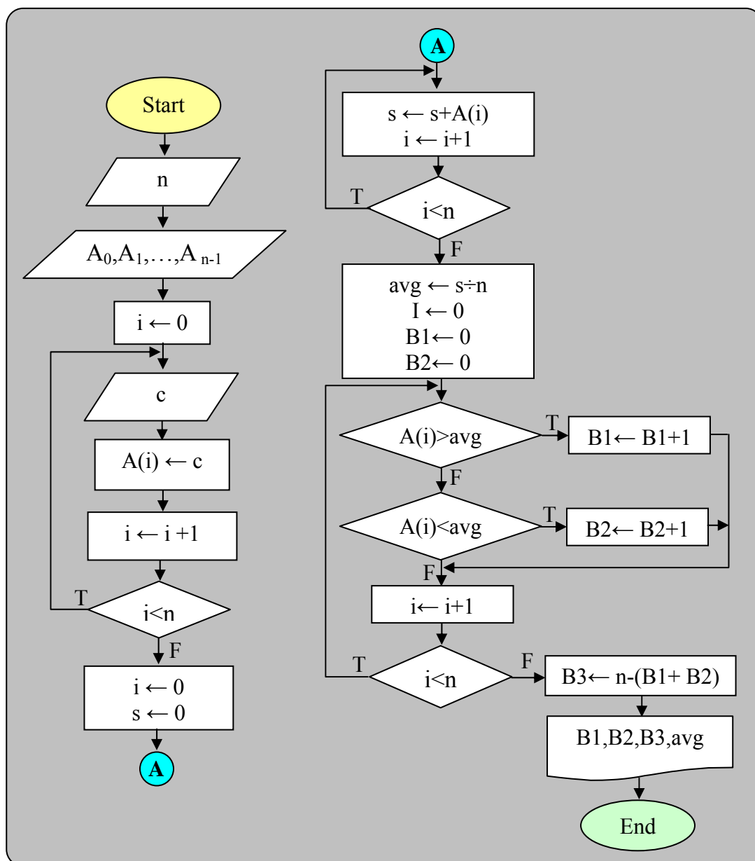
شکل ۲۶: فلوجارت مثال ۱۵
