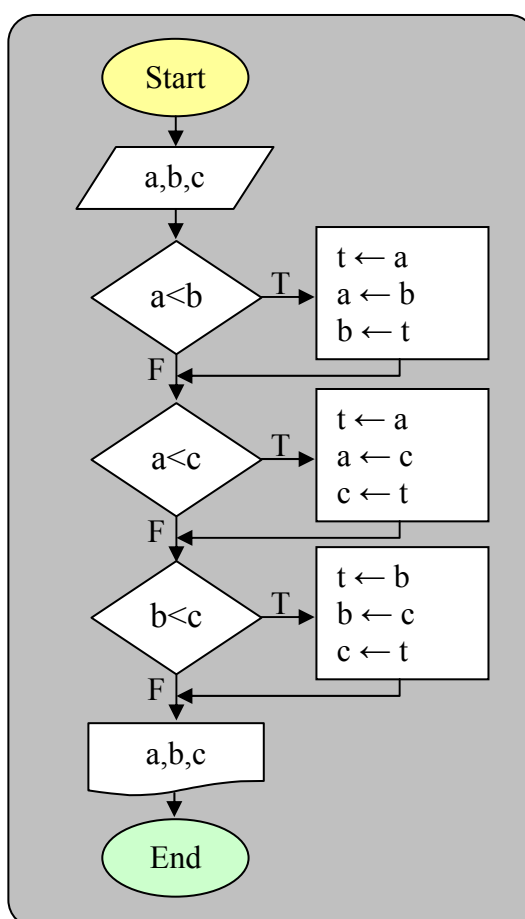
شکل ۱۵: فلوجارت مثال ۶
